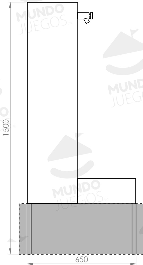
Vista lateral
